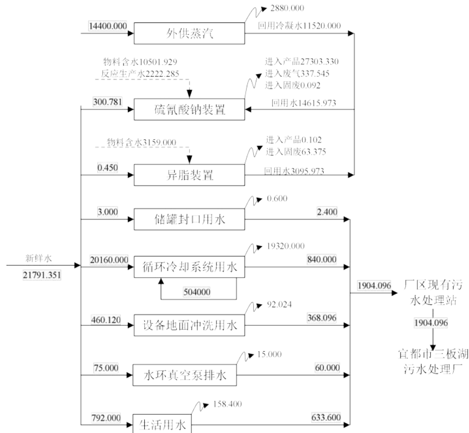
图3-3 项目技改前给排水平衡图
