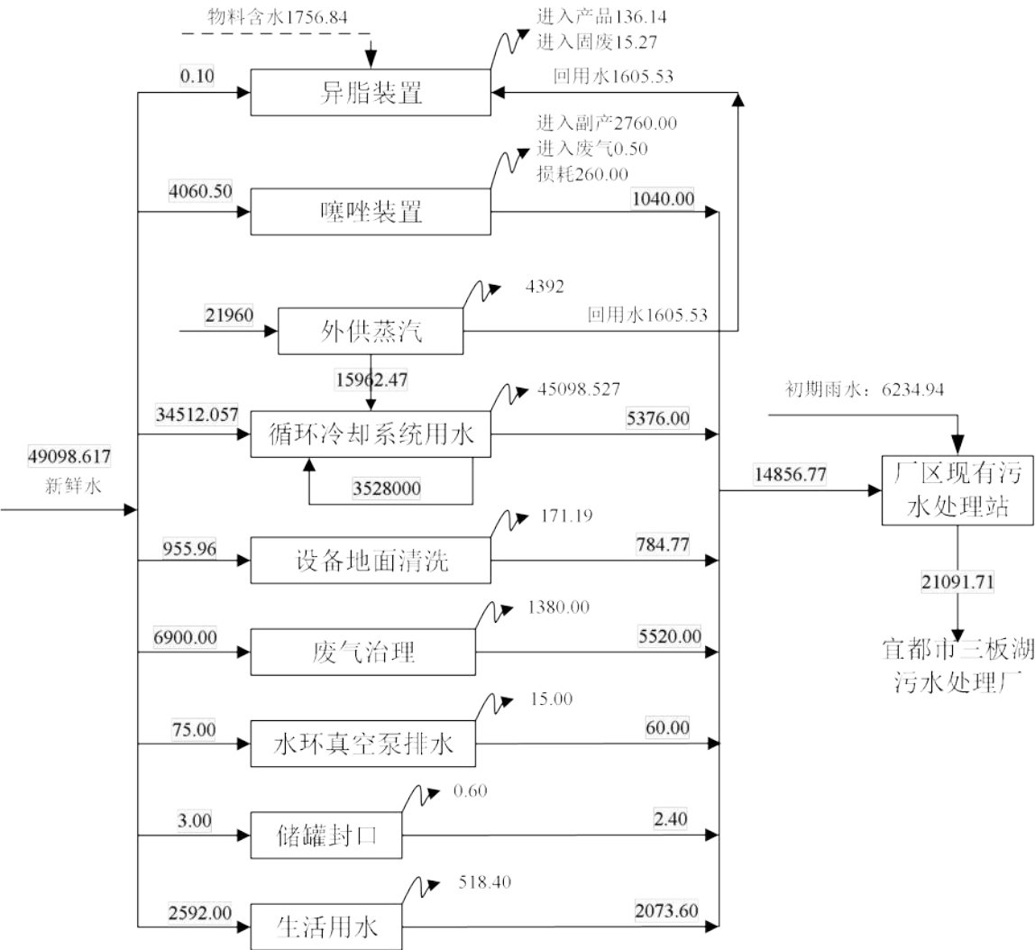
图3-6 全厂给排水平衡图
