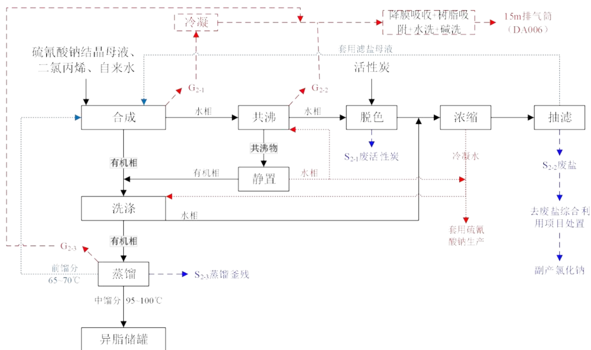
图3-8 硫氰酸钠结晶母液制备异酯工艺流程图
