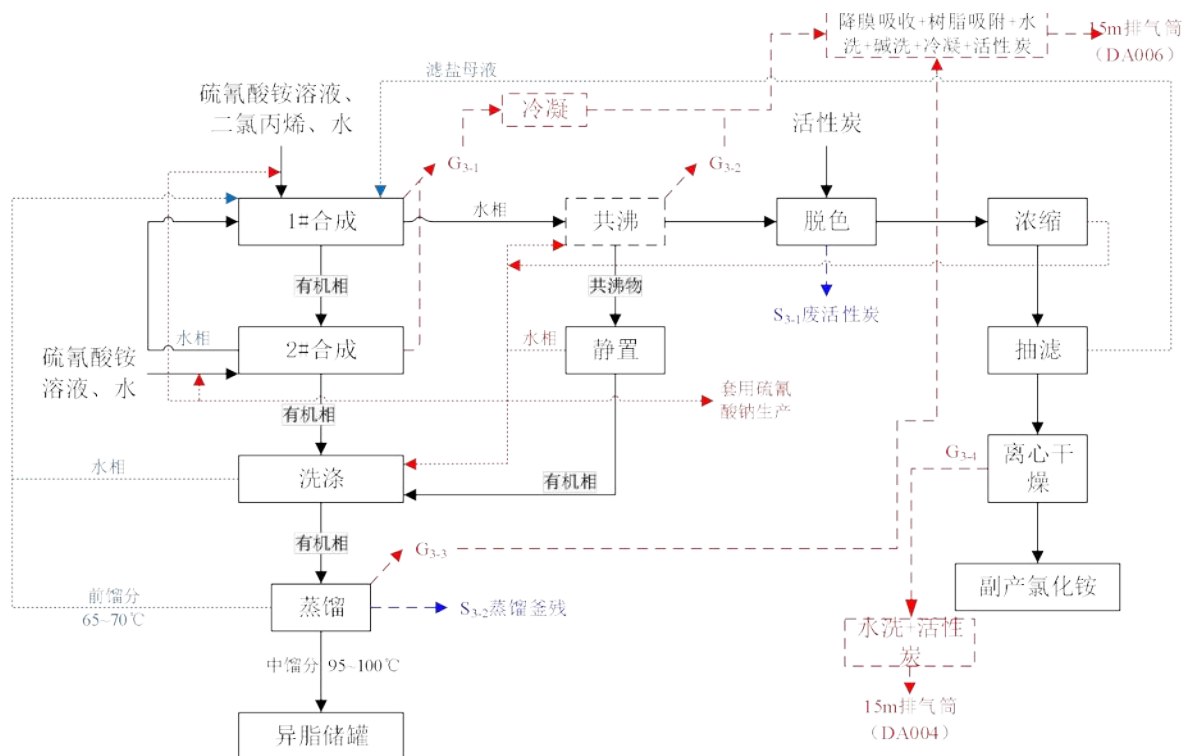
图3-7 硫氰酸铵制备异酯生产线工艺流程图
