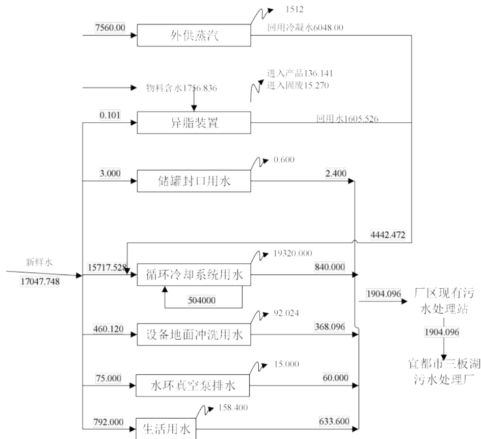
图3-4 项目技改后环评设计给排水平衡图
