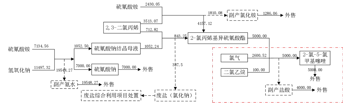
图3-1 羽丰公司技改前企业总体上下游产业路线关系图
